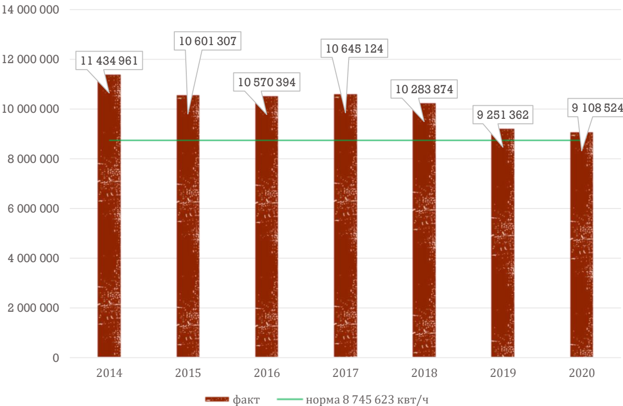
Потребление электроэнергии квт/ч
