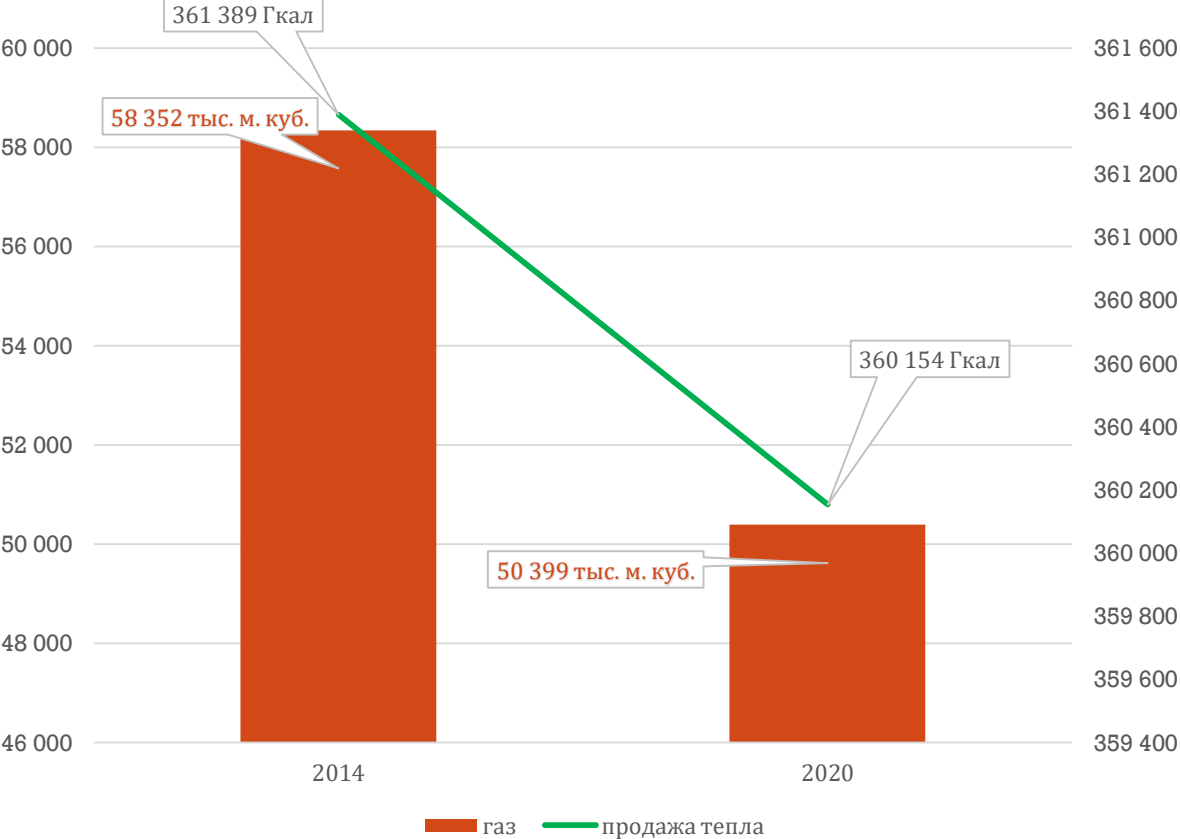
Расход газа и продажа ТЭ
